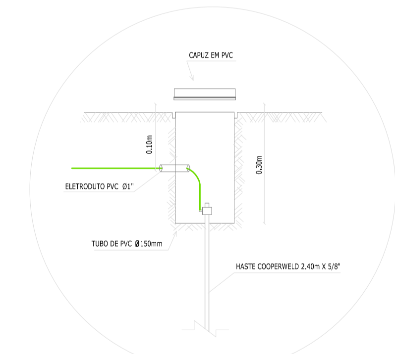
DET. ATERRAMENTO
