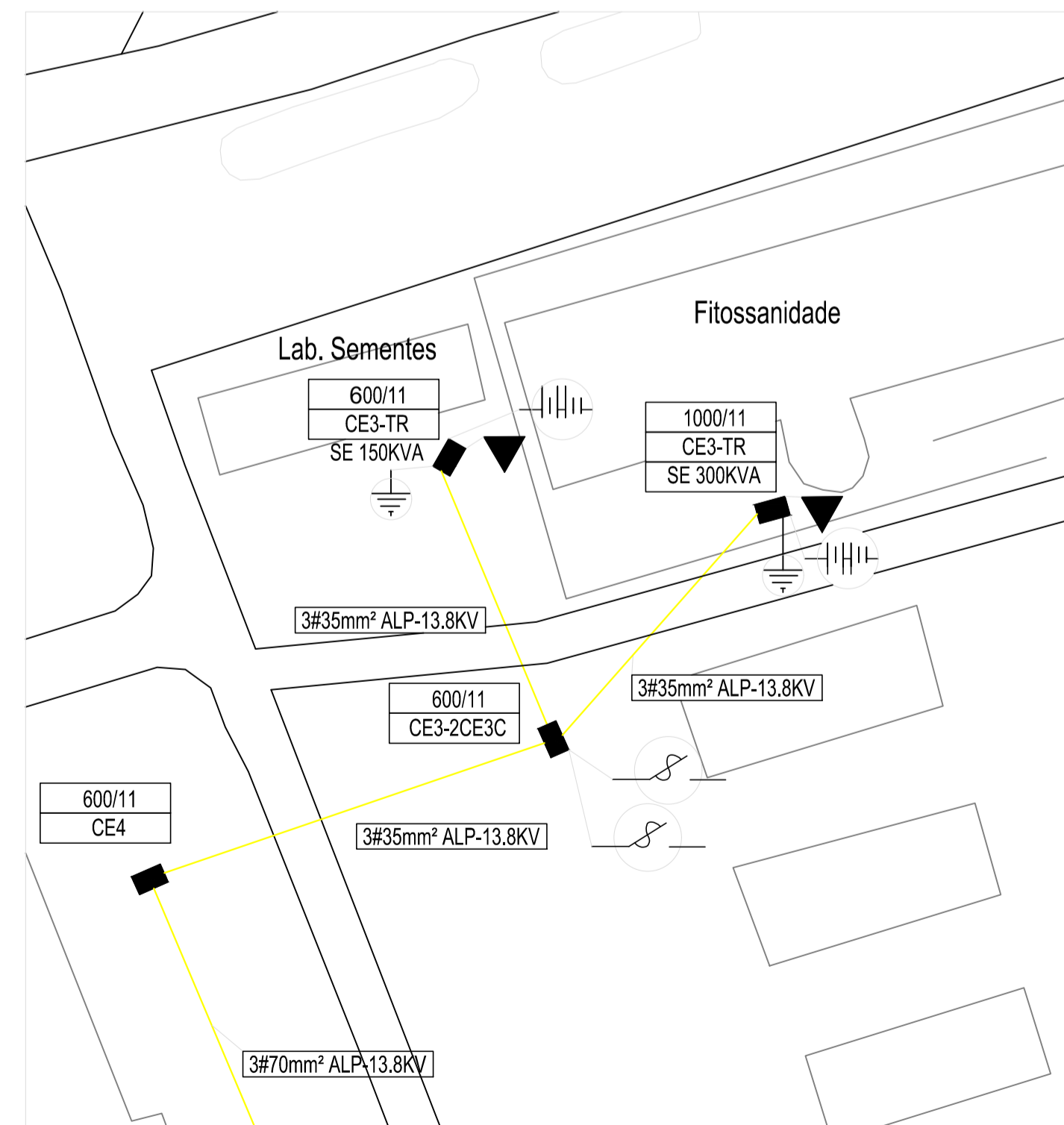
Locação 1/50
