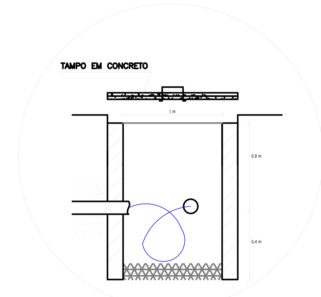
DET. CAIXA DE INSPEÇÃO
